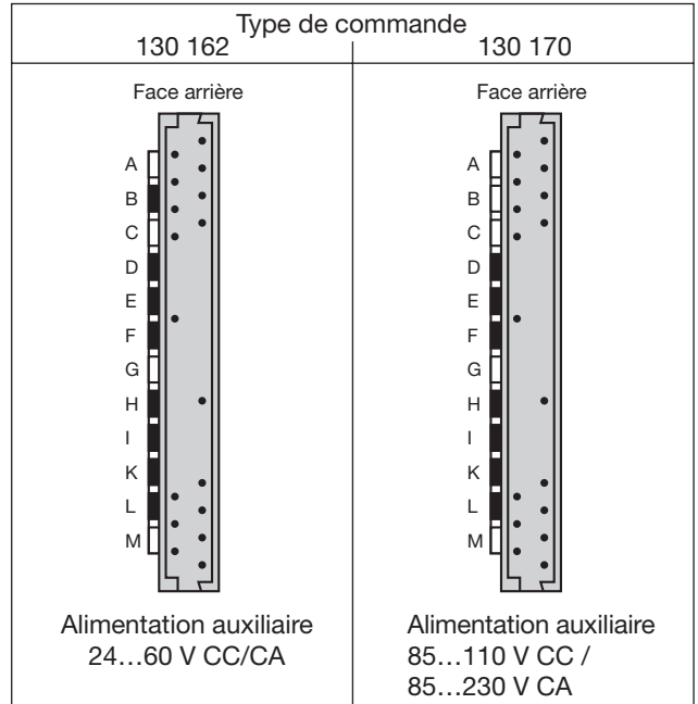
Fig. 4. Codage du module embrochable SIRAX SV 824.
