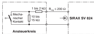
Bild 3. Kontaktbeschaltung.
